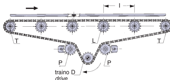
Catena appoggiata Rested chain
